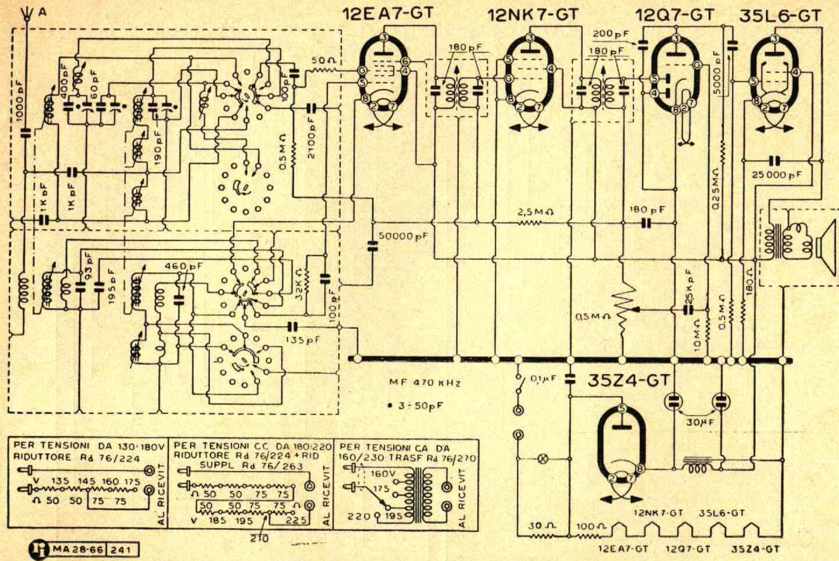
Lo schema elettrico del mod. 9U65/E (*) per i mod. 9U65 e 9U65/C vedere scheda 240
